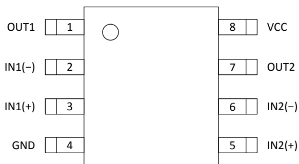
SOP-8 / TSSOP-8
